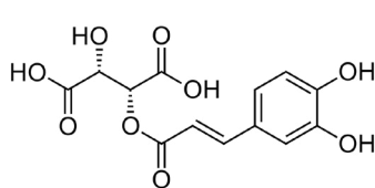
Caftaric acid
